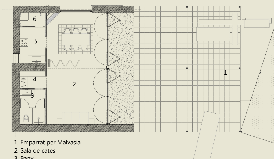
Planta general
