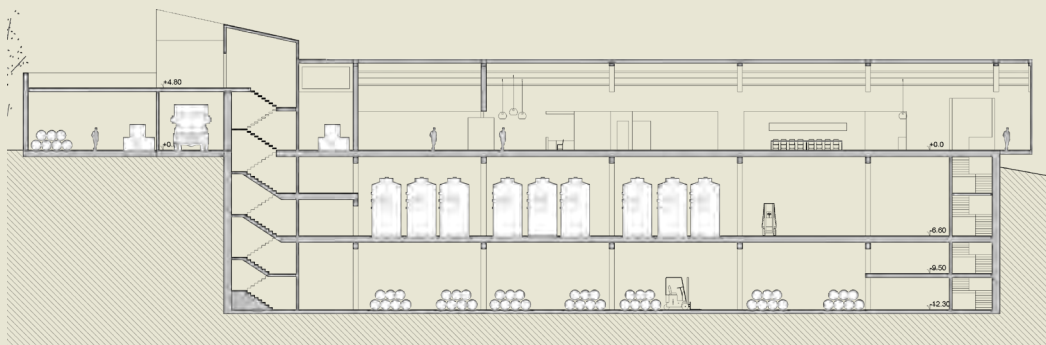
Secció longitudinal
