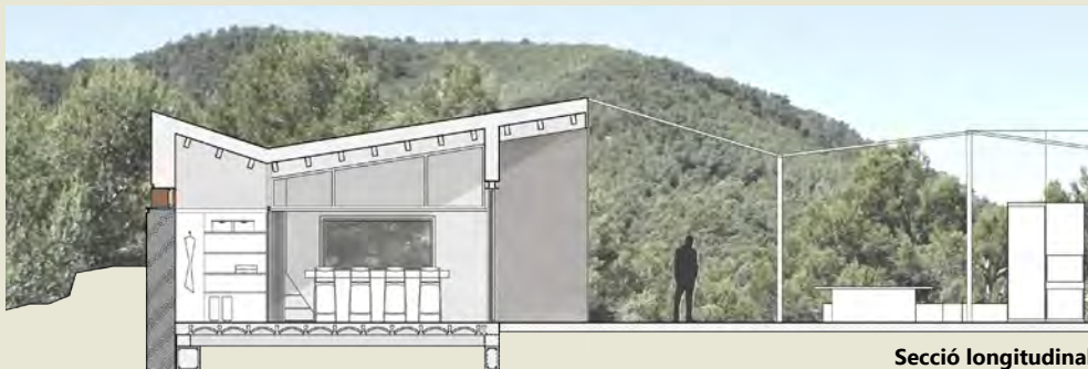
Secció longitudinal
