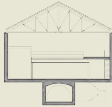
Secció nau principal
